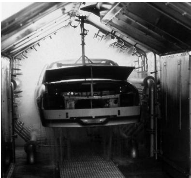
Entfettungs-/Phosphatieranlage
