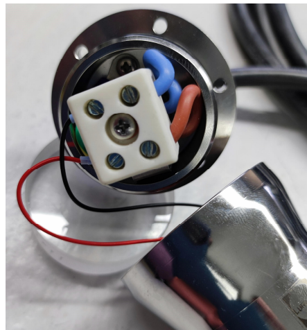
Abbildung 2 Verdrahten
